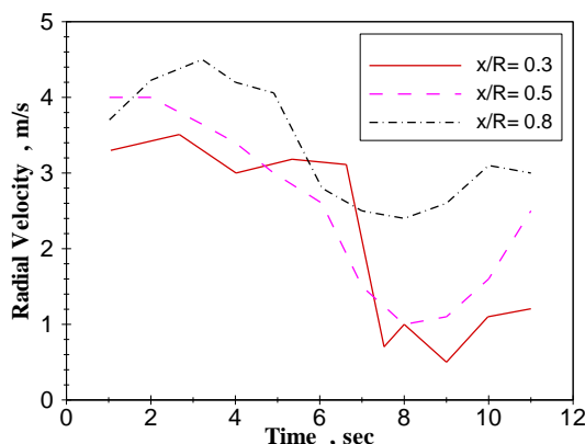
شکل ۱ - تغییرات سرعت شعاعی نسبت به زمان (B Nazanin 10 pt, Bold)
