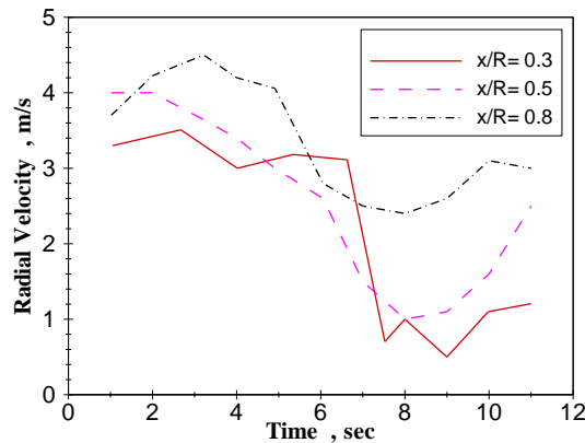
شکل ۱ - تغییرات سرعت شعاعی نسبت به زمان (B Nazanin 10 pt, Bold)
